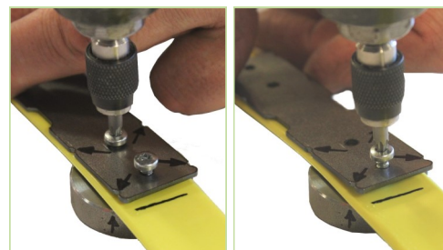
Fest kun ett lodd til klaven og monteringsplata, i enden nærmest klavelåsen.
