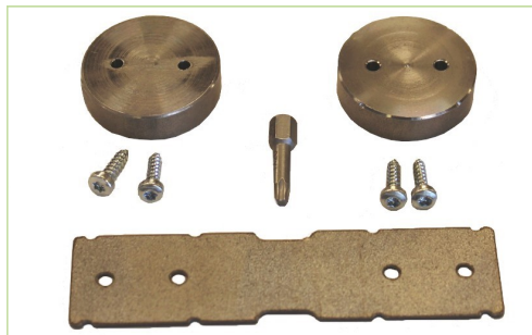
Innhold: lodd, monteringsplate, tilpasset bit og skruer.
